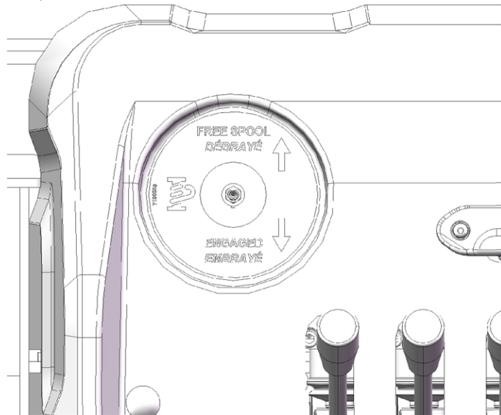
FIGURE 5 – COMMANDE DE DÉBRAYAGE DES TREUILS
