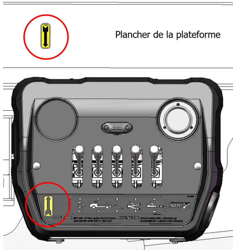
FIGURE 18 – GLISSER LE PLANCHER VERS L'ARRIÈRE
