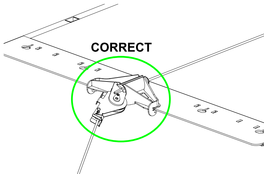
FIGURE 76 – UTILISATION CORRECTE D'UNE POULIE
