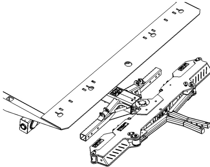
FIGURE 95 – LÈVE-ROUES À CHARGEMENT AUTOMATIQUE AVEC SES BRAS EN L OUVERTS
