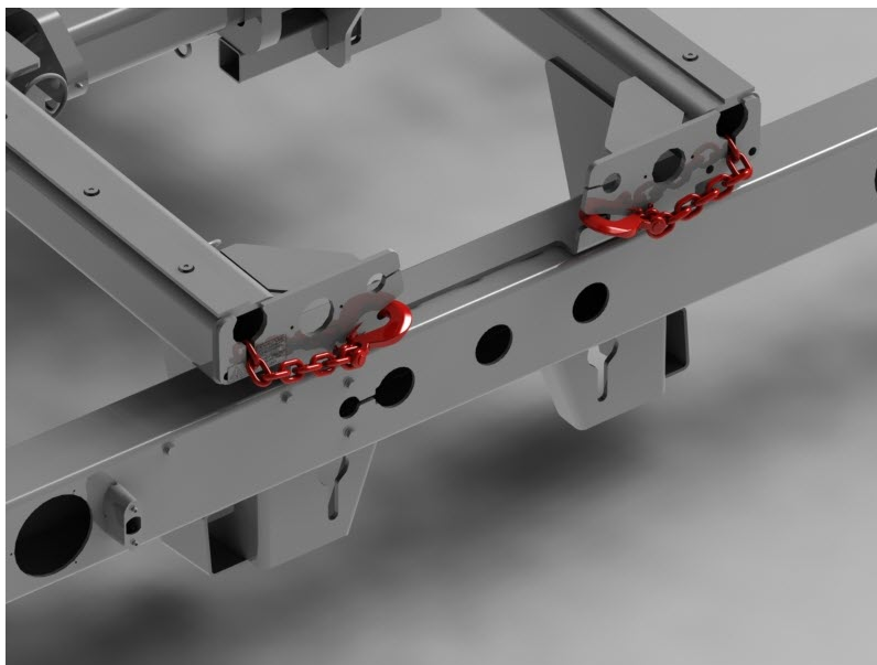
FIGURE 105 – CHÂÎNES DE SÉCURITÉ RÉTRACTABLES
