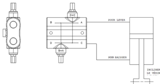
FIGURE 40 – AJUSTEMENT DE LA SOUPAPE D'AMORTISSEMENT DU BRAS DE REMORQUAGE
