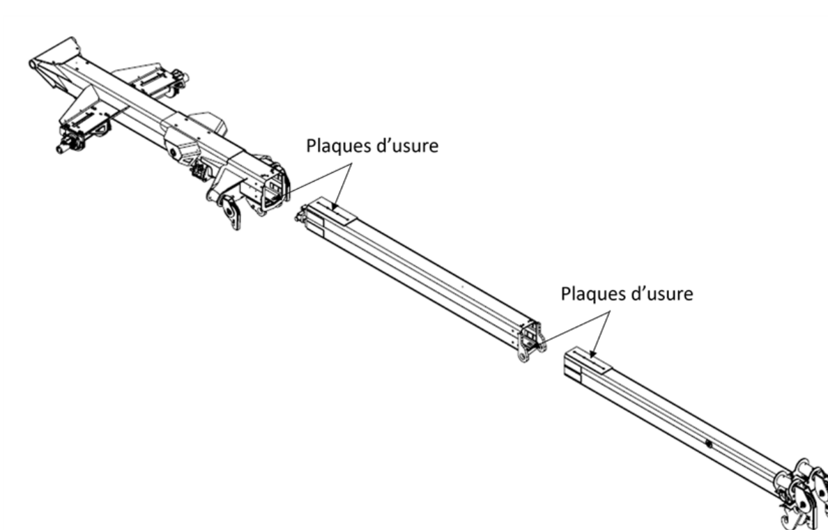
FIGURE 32 – PLAQUES D'USURE – FLÈCHE
