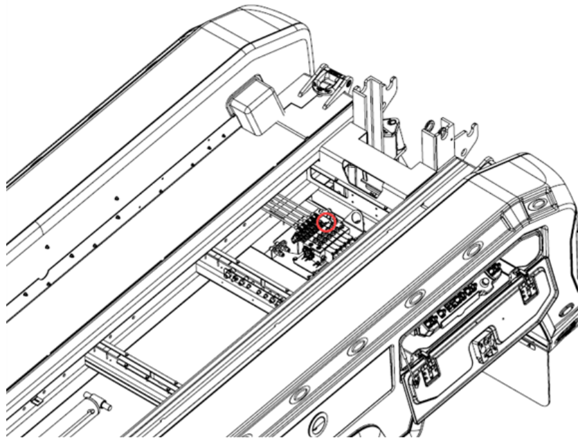
FIGURE 37 – EMBLACEMENT DE LA VIS D'AJUSTEMENT DE LA SOUPAPE SOUS LE PLANCHER DE LA DÉPANNÉUSE
