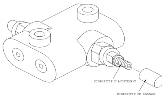
FIGURE 41 – AJUSTEMENT DE LA SOUPAPE D'AMORTISSEMENT
