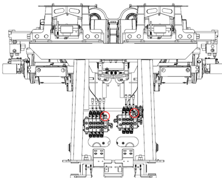
FIGURE 36 – EMPLACEMENT DES VIS D'AJUSTEMENT DES SOUPAPES DANS LA BASE DE LA FLÈCHE
