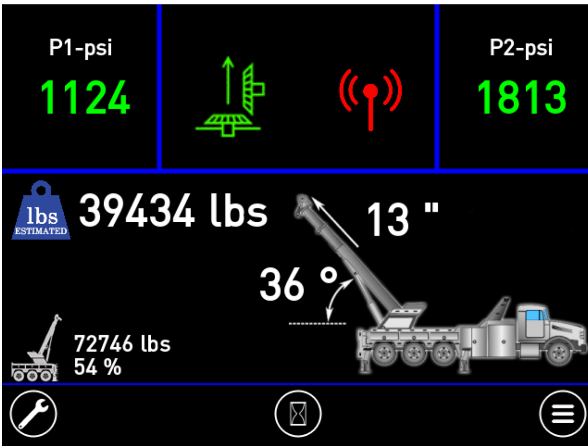
FIGURE 6 — ÉCRAN (EXEMPLE)
