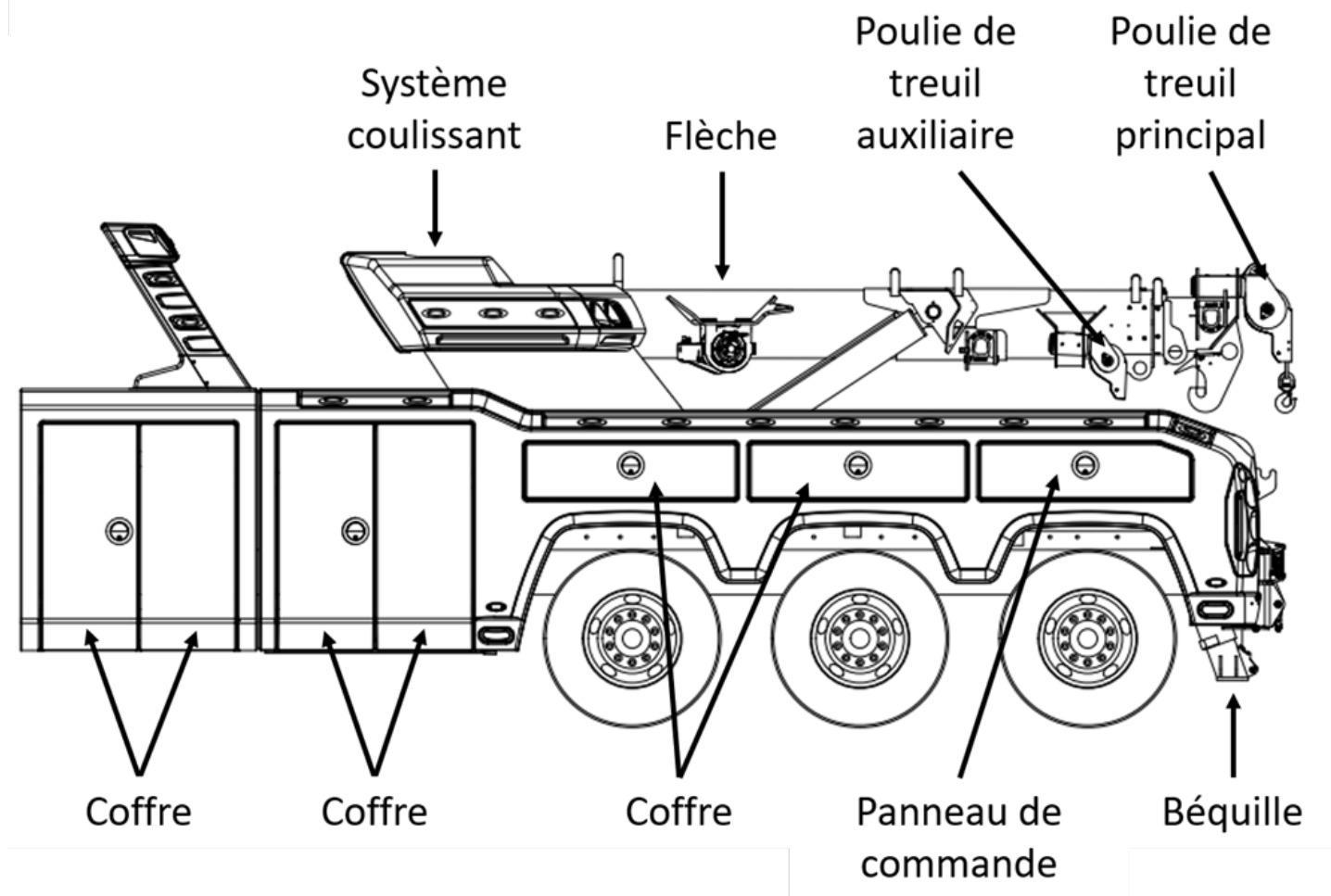
FIGURE 1 — CHÂSSIS SANS BRAS DE REMORQUAGE (EXEMPLE)
