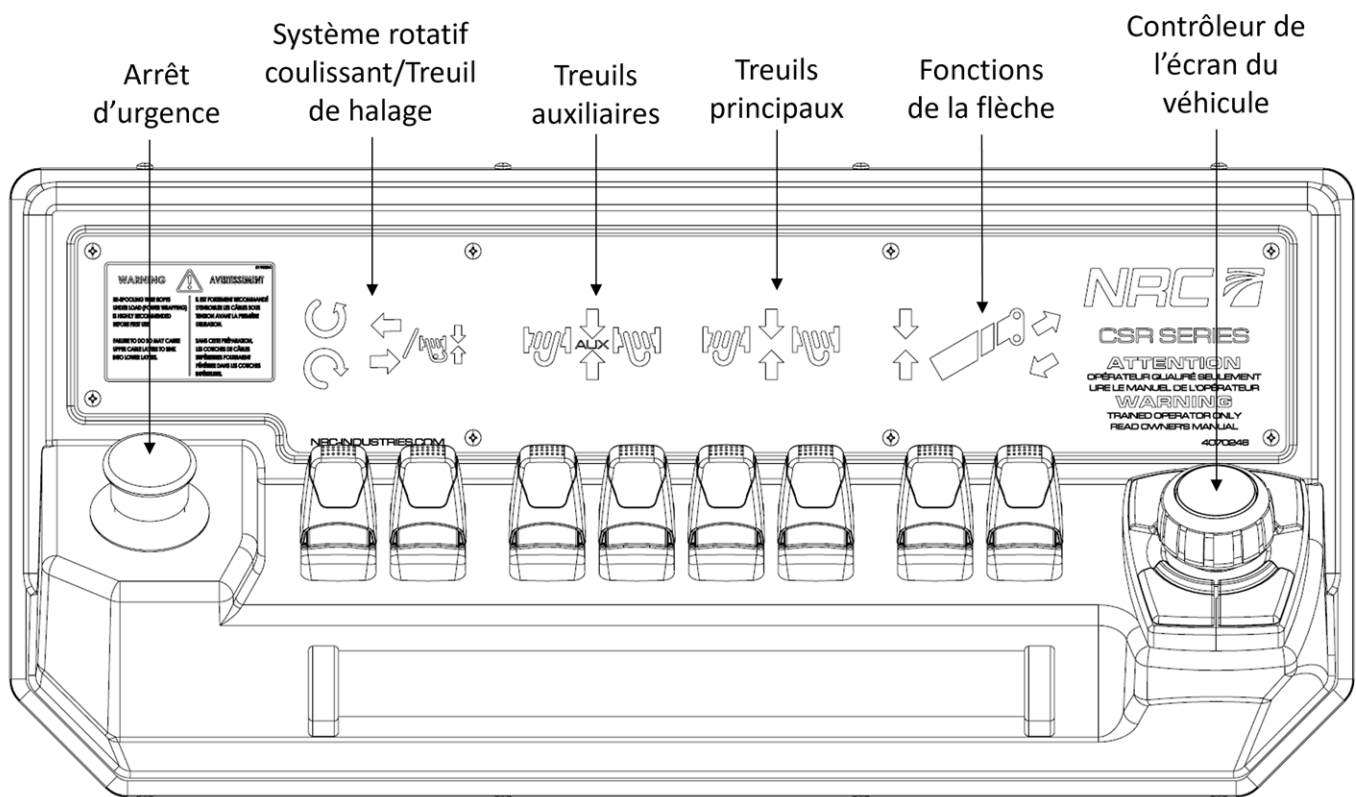
FIGURE 6 – PANNEAU DE COMMANDE (EXEMPLE)
