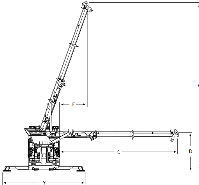
FIGURE 14 – DIMENSIONS DE LA FLÈCHE ET DES STABILISATEURS - VUE ARRIÈRE (EXEMPLE)
