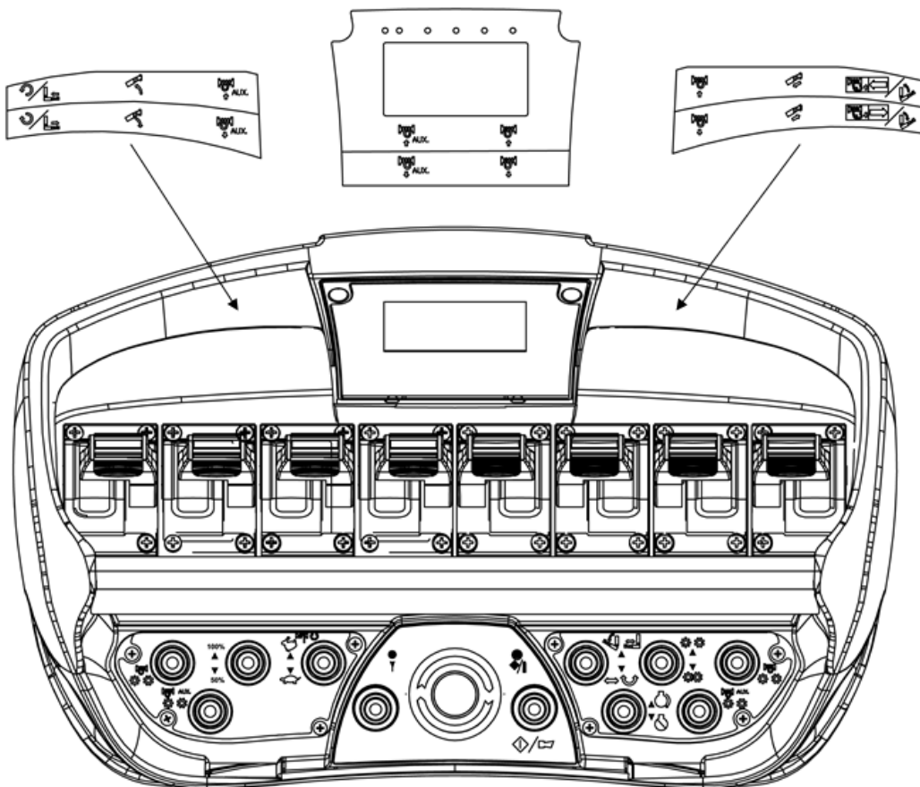
FIGURE 10 – TÉLÉCOMMANDE (EXEMPLE)
