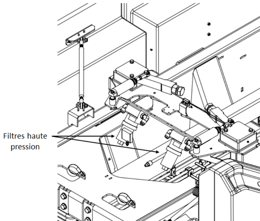
FIGURE 38 – FILTRES À HAUTE PRESSION – CSR50
