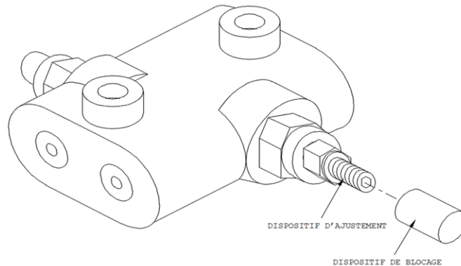
FIGURE 55 – AJUSTEMENT DE LA SOUPE D'AMORTISSEMENT
