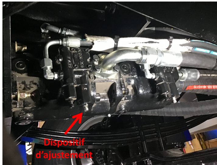
FIGURE 42 – EMPLACEMENT DE LA VIS POUR L'AJUSTEMENT DE LA PRESSION DE LA POMPE HYDRAULIQUE (CSR50 ET CSR65)
