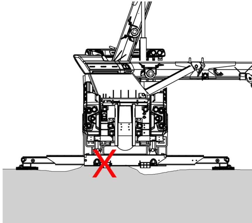
FIGURE 18 – STABILISATEURS TOUCHANT LE SOL (EXEMPLE)
