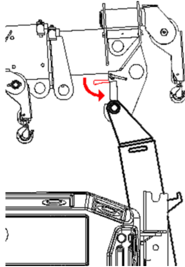
FIGURE 23 – DÉVERROUILLER L'ATTACHE DE SÉCURITÉ (EXEMPLE)
