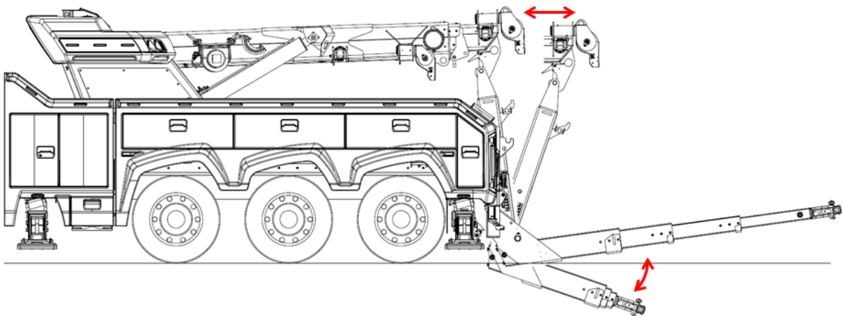
FIGURE 21 – MOUVEMENTS DU BRAS DE REMORQUAGE
