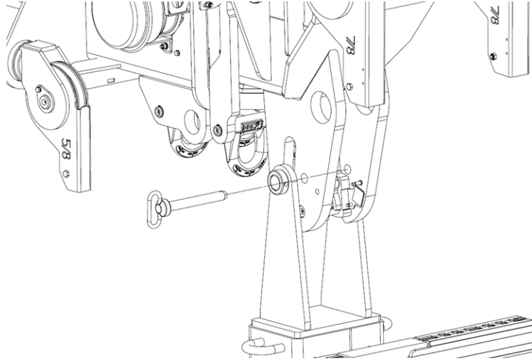
FIGURE 24 – ENLEVER LA GOUPILLE DE SÉCURITÉ
