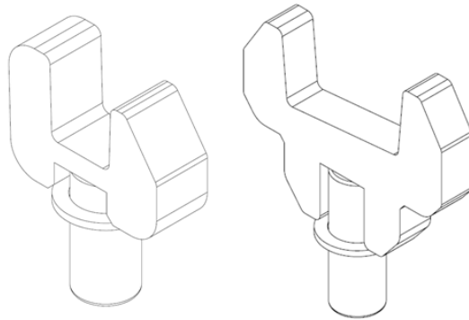
FIGURE 58 – EXEMPLE DE FOURCHES
