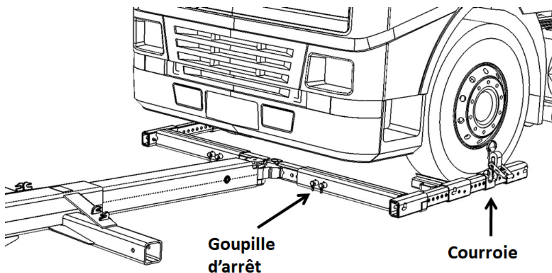
FIGURE 69 – INSTALLER LES LÈVE-PNEUS POUR VÉHICULES DE POIDS MOYEN
