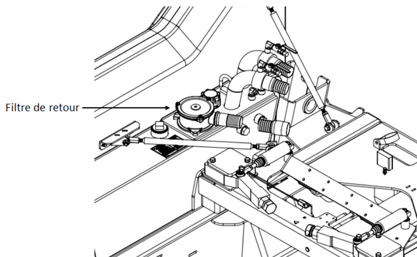
FIGURE 39 – FILTRE DE RETOUR – CSR50
