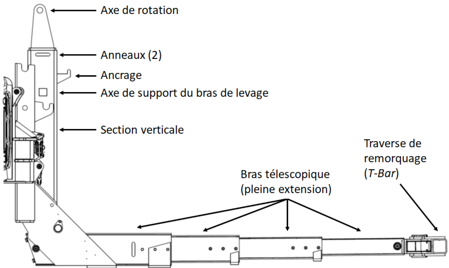
FIGURE 4 – BRAS DE REMORQUAGE (EXEMPLE)
