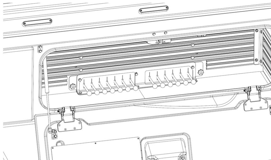
FIGURE 19 – DÉRIVATION HYDRAULIQUE D'URGENCE DANS L'ARMOIRE
