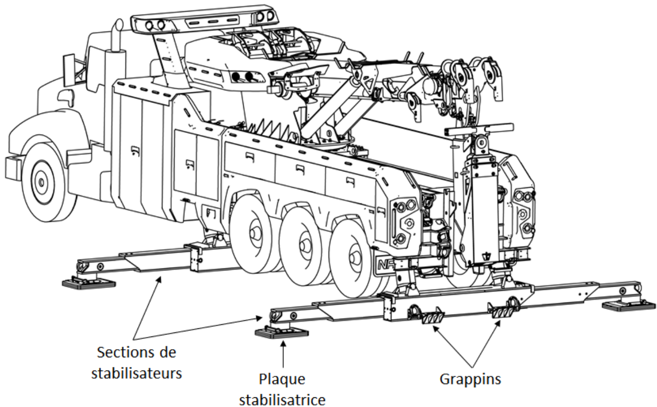
FIGURE 2 – STABILISATEURS (EXEMPLE)
