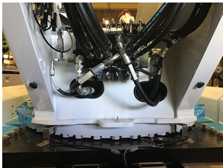
FIGURE 47 – EMBLACEMENT DU DISTRIBUTEUR DANS LA BASE DE LA FLÈCHE (CSR85)
