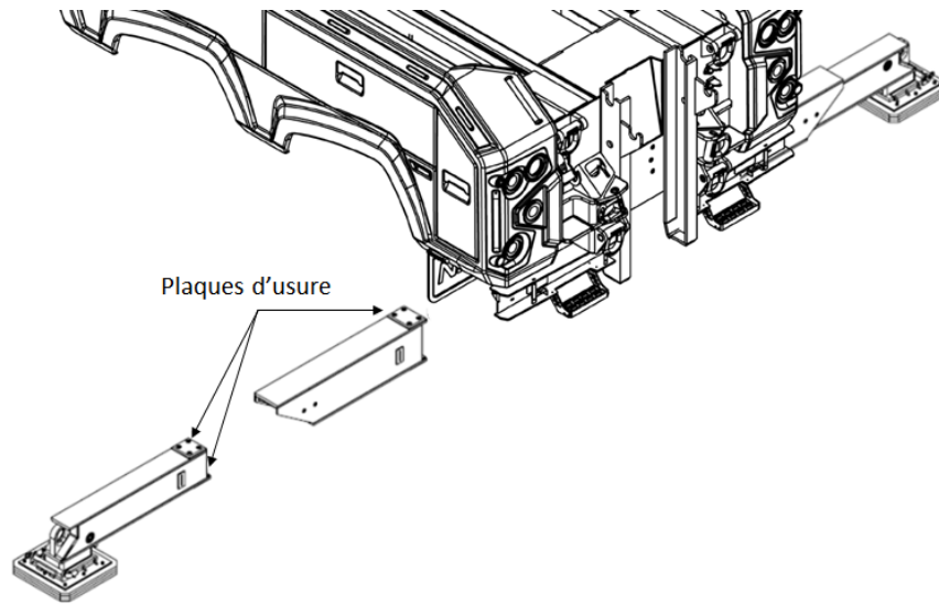
FIGURE 34 – PLAQUES D'USURE – STABILISATEURS
