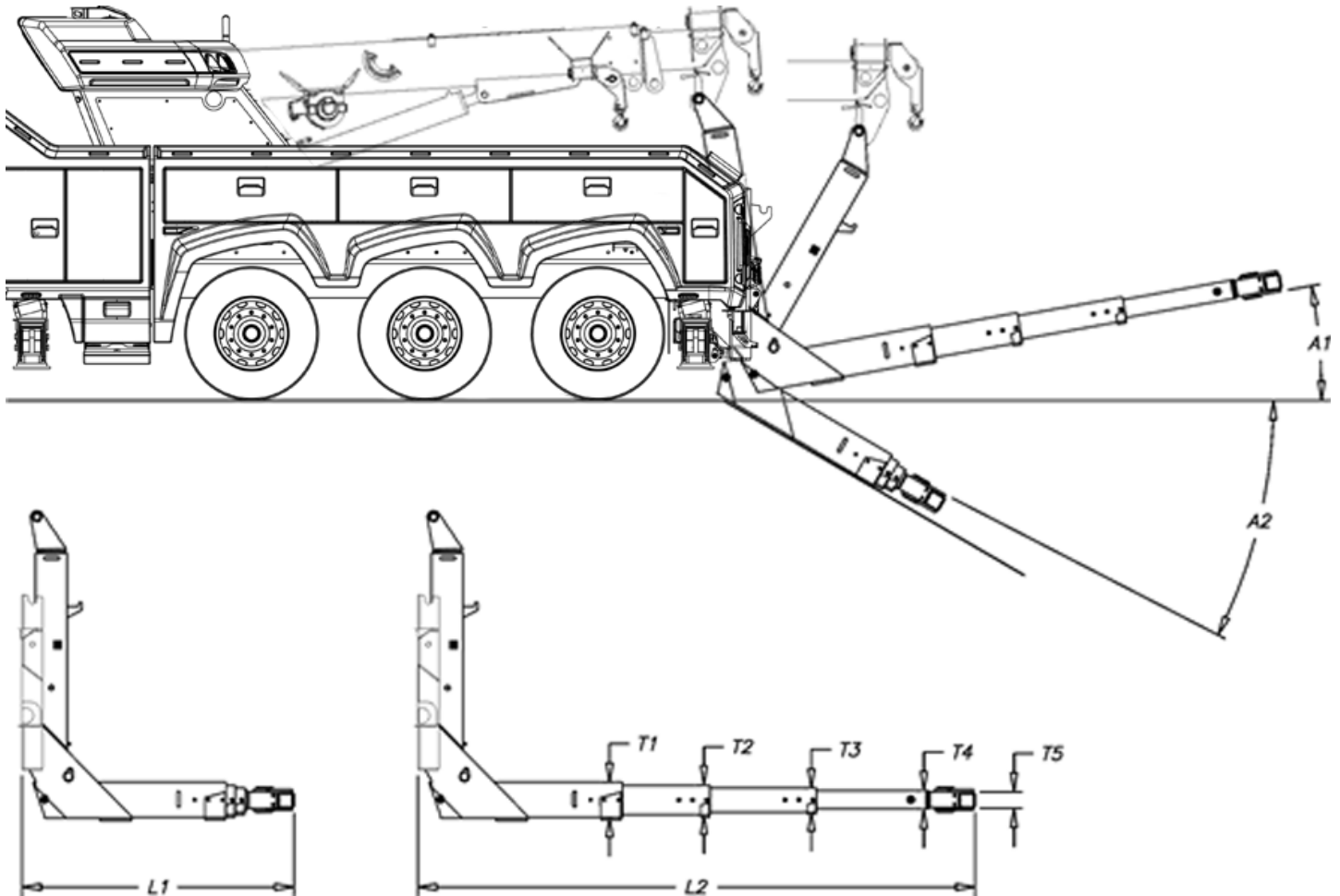
FIGURE 16 - DIMENSIONS DU BRAS DE REMORQUAGE (EXEMPLE)
