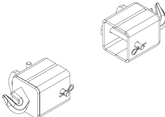
FIGURE 63 – EXEMPLE DE SUPPORTS DE TRAVERSES DE REMORQUAGE
