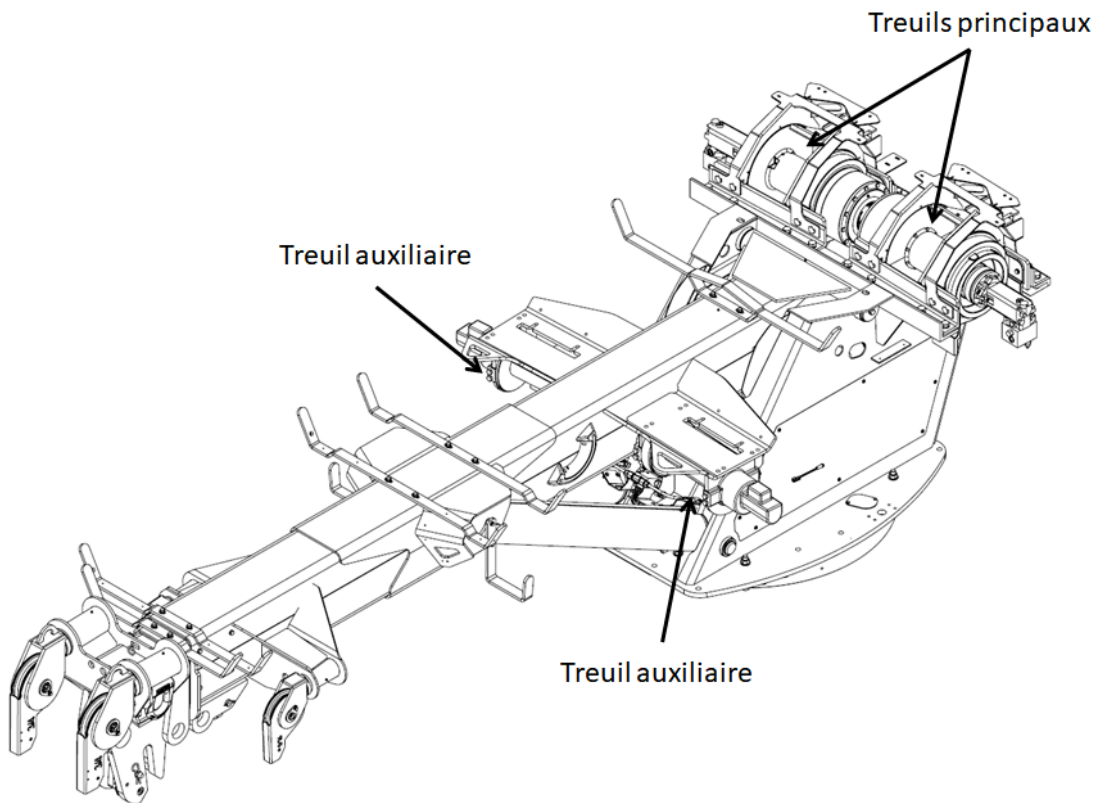
FIGURE 31 – EMPLACEMENT DES TREUILS
