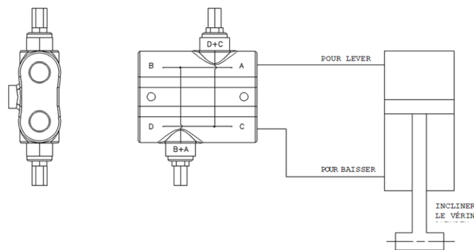
FIGURE 54 – AJUSTEMENT DE LA SOUPAPE D'AMORTISSEMENT DU BRAS DE REMORQUAGE
