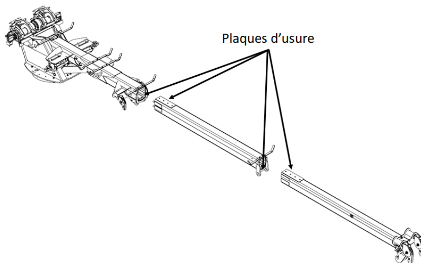
FIGURE 33 – PLAQUES D'USURE – FLÈCHE
