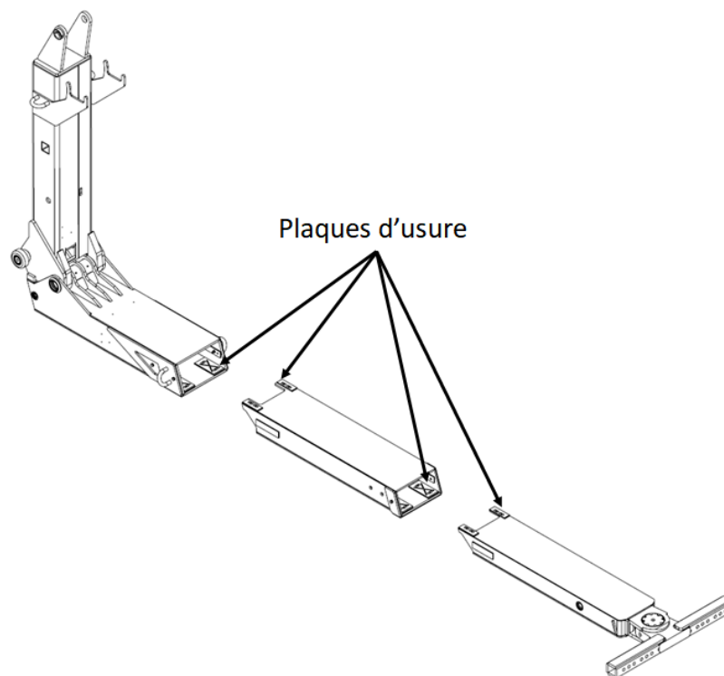
FIGURE 32 – PLAQUES D'USURE – BRAS DE REMORQUAGE
