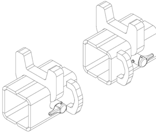
FIGURE 61 – EXEMPLE DE SUPPORTS À FOURCHES INTÉGRÉES
