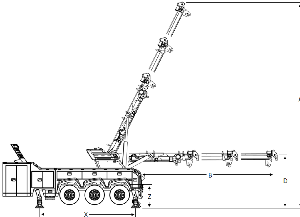
FIGURE 13 – DIMENSIONS DE LA FLÈCHE ET DES STABILISATEURS - VUE LATÉRALE (EXEMPLE)
