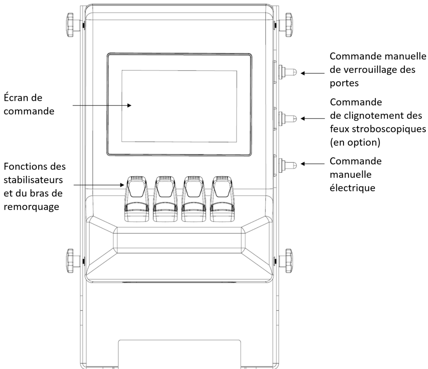
FIGURE 7 – PANNEAU D'ÉCRAN MD4-7, FERMÉ (EXEMPLE)
