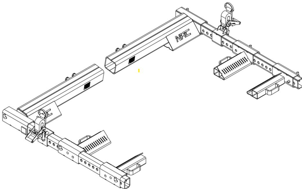
FIGURE 68 – EXEMPLE DE LÈVE-PNEUS POUR VÉHICULES DE POIDS MOYEN
