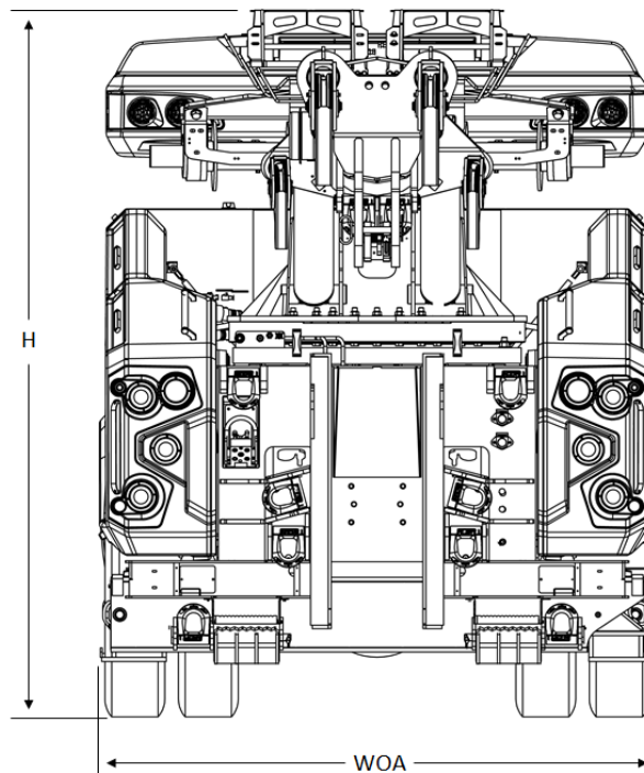
FIGURE 12 – DIMENSIONS DU CHÂSSIS - VUE DE DESSUS (EXEMPLE)
