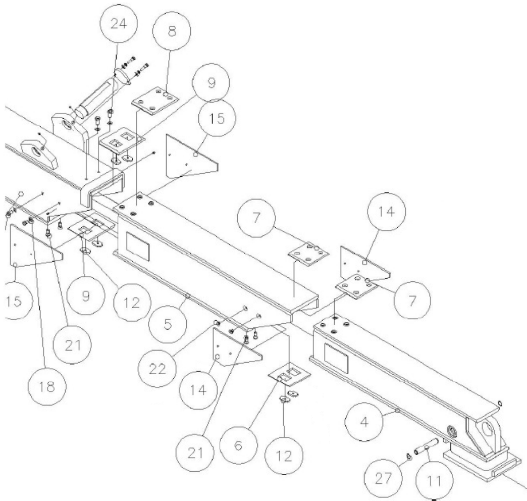
FIGURE 56 – DÉMONTER LE STABILISATEUR (CSR50)
