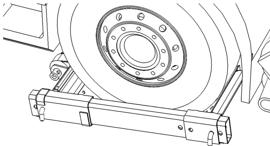
FIGURE 67 – INSTALLER LES COURROIES
