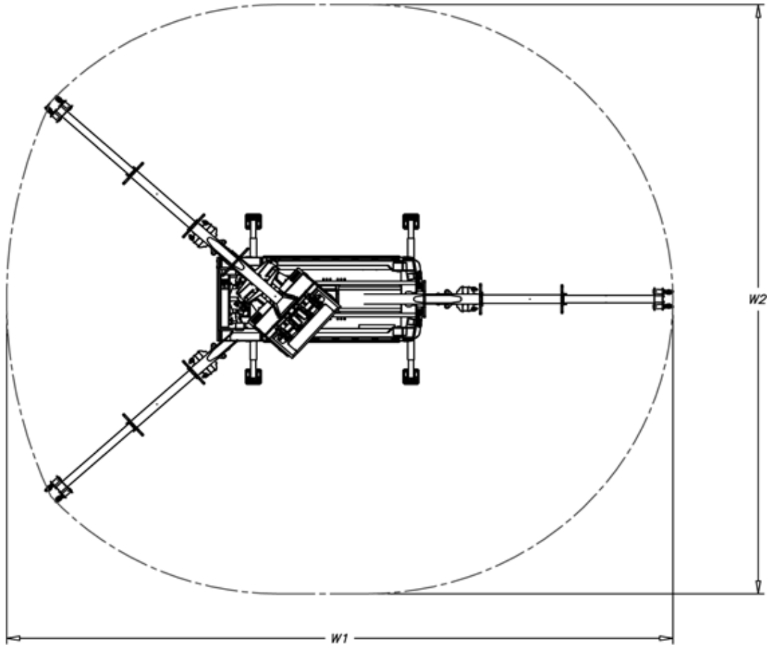
FIGURE 15 – DIMENSIONS DE LA ZONE DE TRAVAIL - VUE DE DESSUS (EXEMPLE)
