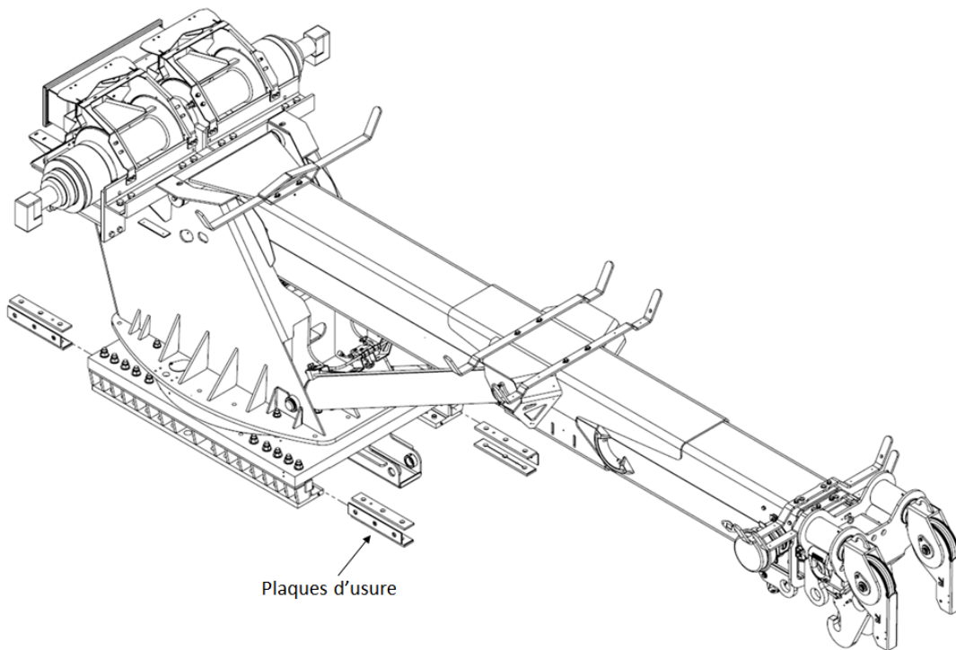
FIGURE 35 – PLAQUES D'USURE – SYSTÈME COULISSANT
