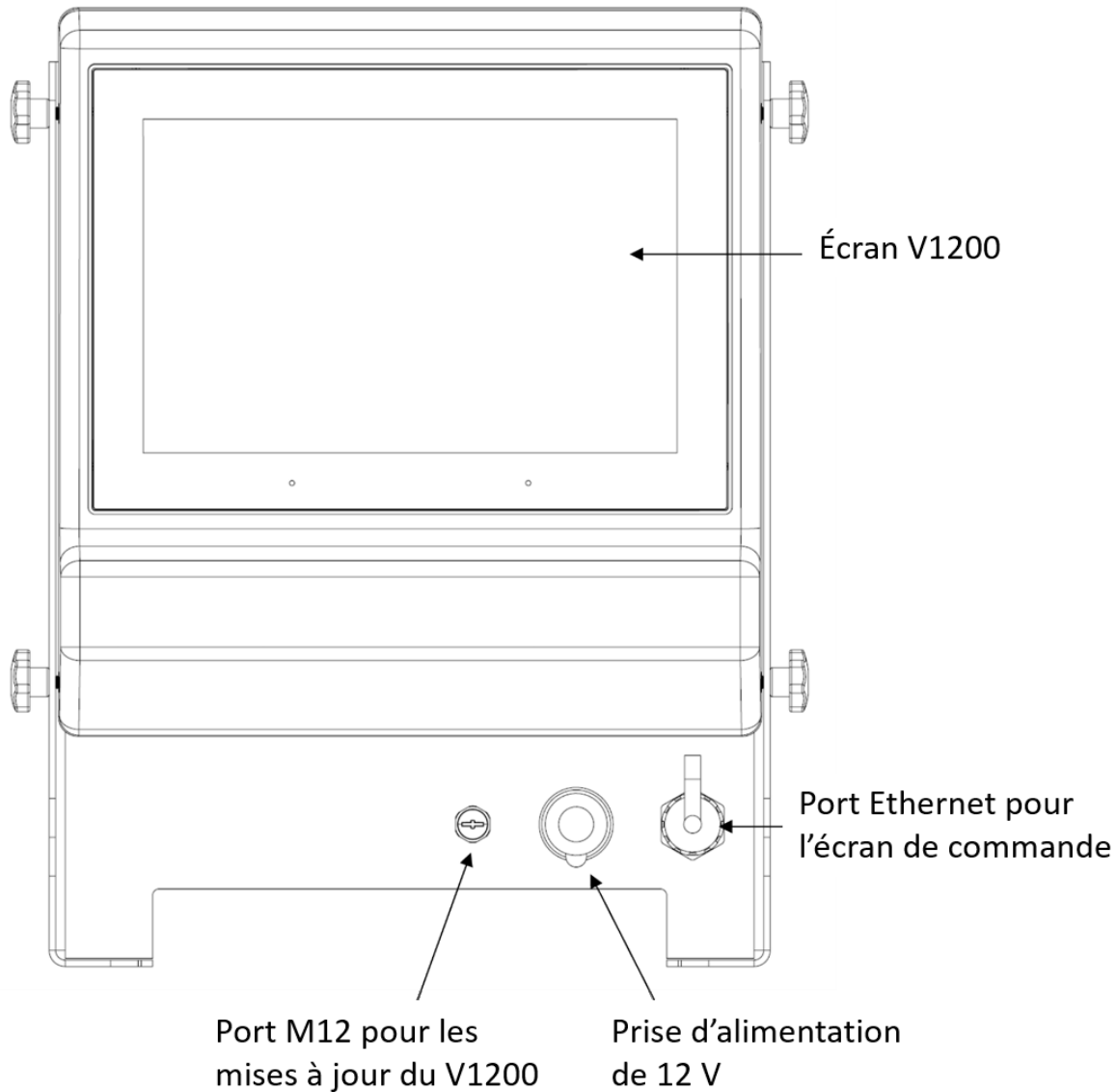
FIGURE 9 – PANNEAU D'ÉCRAN V1200 (EXEMPLE)
