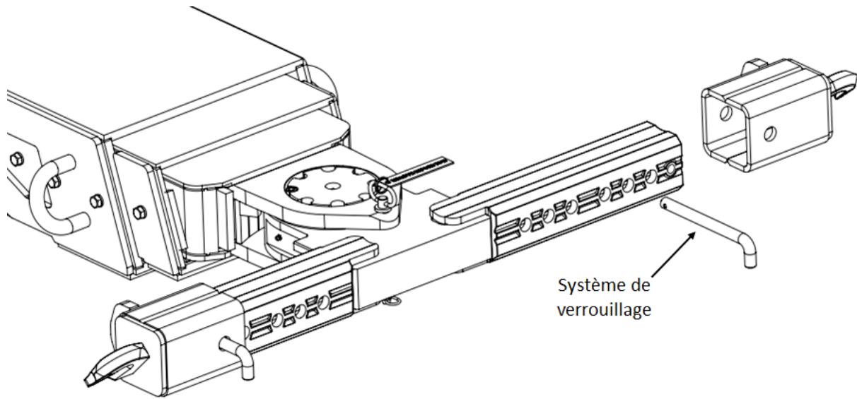
FIGURE 64 – INSTALLER LES SUPPORTS DE TRAVERSES DE REMORQUAGE
