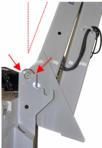
FIGURE 27 – PLACER LE BRAS DE REMORQUAGE DANS LES RAILS (EXEMPLE)
