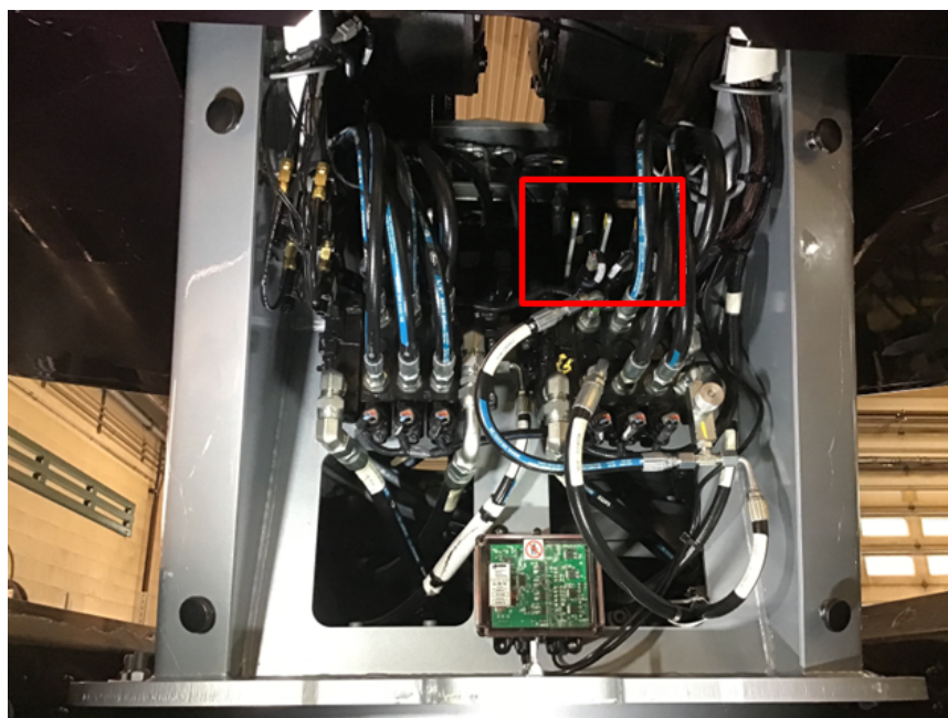
FIGURE 20 – DÉRIVATION HYDRAULIQUE D'URGENCE DANS LA BASE DU SYSTÈME COULISSANT ROTATIF
