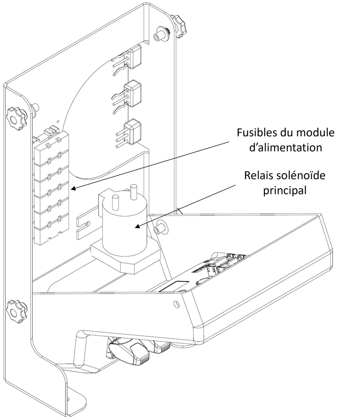
FIGURE 8 – PANNEAU D'ÉCRAN MD4-7, OUVERT (EXEMPLE)
