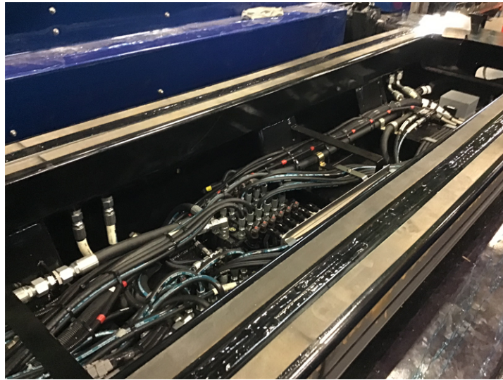
FIGURE 44 – EMBLACEMENT DES DISTRIBUTEURS À L'INTÉRIEUR DE LA CARROSSERIE DE LA DÉPANNEUSE (CSR50 ET CSR65)
