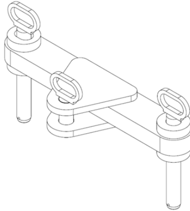
FIGURE 72 – EXEMPLE D'ADAPTATEUR POUR BARRE DE REMORQUAGE
