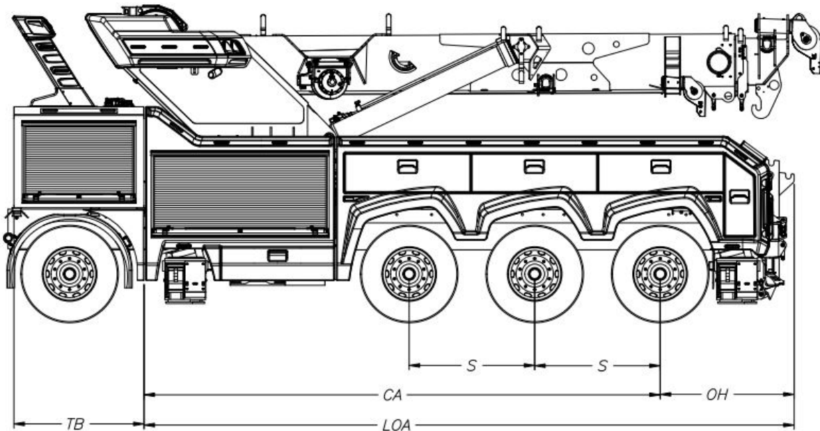
FIGURE 11 – DIMENSIONS DU CHÂSSIS - VUE LATÉRALE (MODÈLE CSR85 ILLUSTRÉ)
