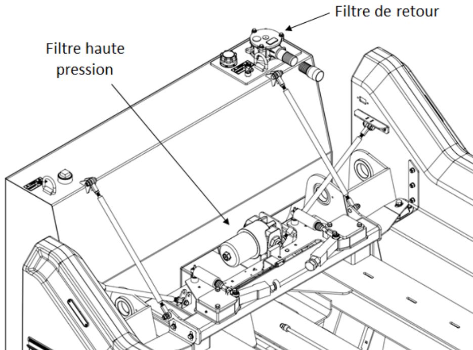
FIGURE 41 – FILTRES POUR LE MODÈLE - CSR85
