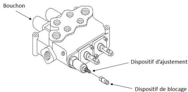
FIGURE 45 – AJUSTER LA PRESSION HYDRAULIQUE SUR LES MODÈLES CSR50 ET CSR65 (SOUPAPE DE SURPRESSION PRINCIPALE)
