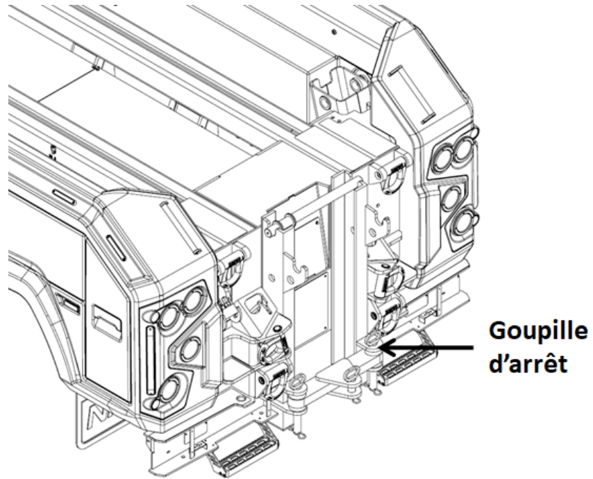
FIGURE 73 – INSTALLER L'ADAPTATEUR POUR BARRE DE REMORQUAGE
