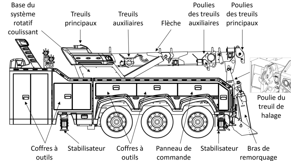
FIGURE 1 – COMPOSANTS DU CHÂSSIS ET DE LA DÉPANNEUSE (EXEMPLE)
