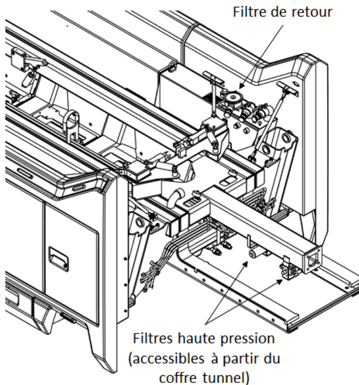
FIGURE 40 – FILTRES POUR LE MODÈLE - CSR65
