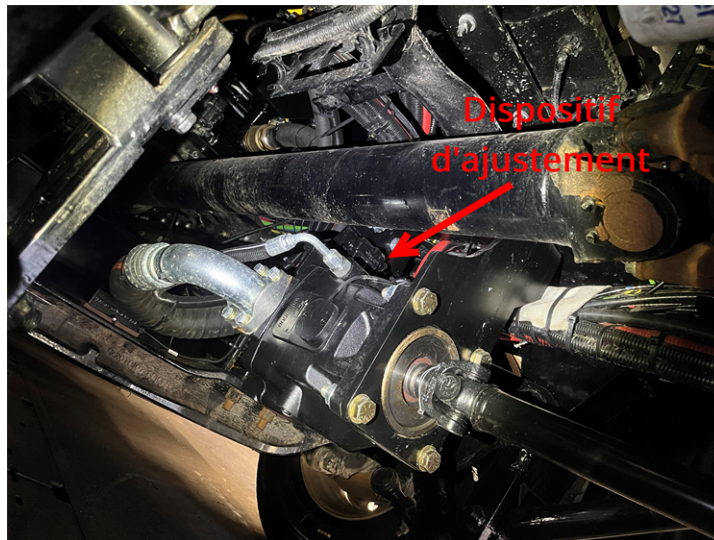
FIGURE 46 – EMBLACEMENT DE LA VIS POUR L'AJUSTEMENT DE LA PRESSION DE LA POMPE HYDRAULIQUE (CSR85)
