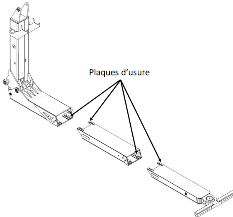
FIGURE 36 – PLAQUES D'USURE – BRAS DE REMORQUAGE
