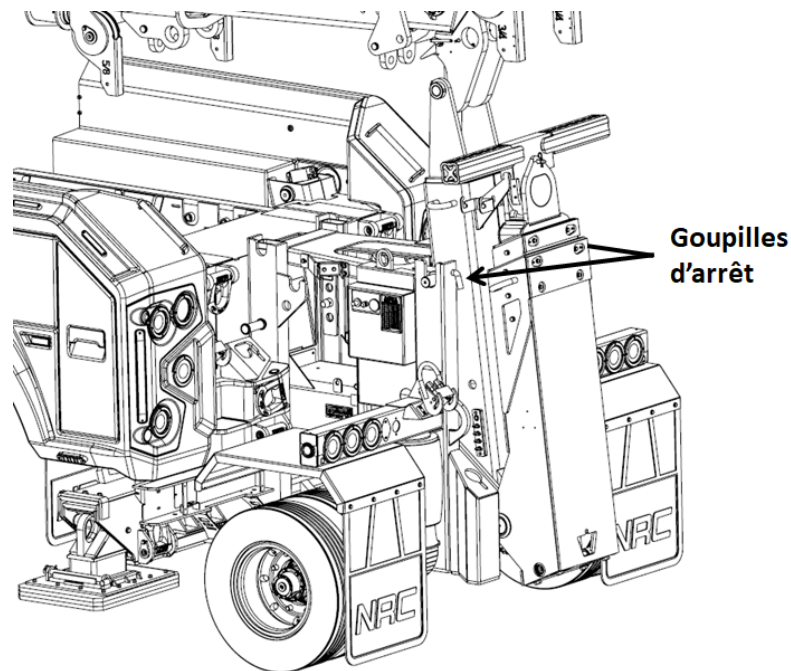
FIGURE 33 – FIXER LE BRAS DE REMORQUAGE À L'ESSIEU D'APPOINT
