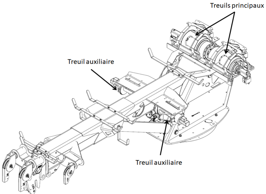
FIGURE 35 – EMBLACEMENT DES TREUILS
