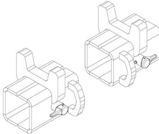
FIGURE 65 – EXEMPLE DE SUPPORTS À FOURCHES INTÉGRÉES
