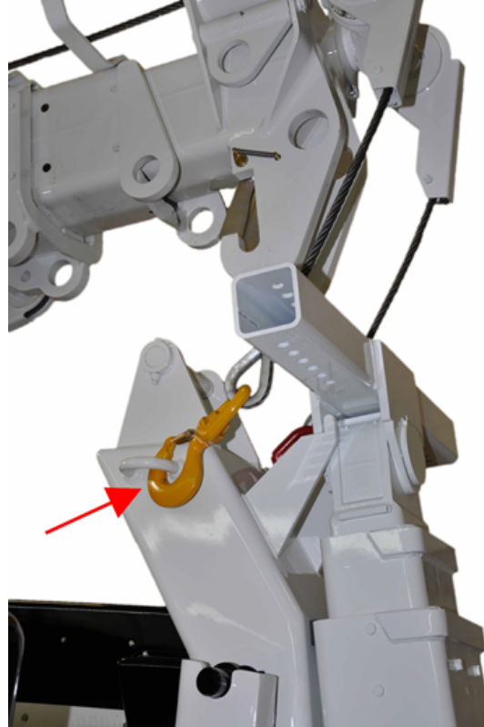
FIGURE 30 – FIXER LES CÂBLES AUX ŒILLETS (EXEMPLE)
