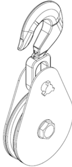
FIGURE 75 – EXEMPLE D'UNE POULIE COUPÉE
