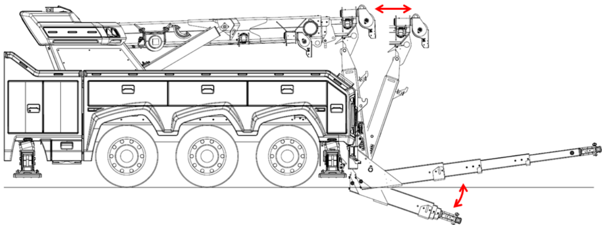
FIGURE 25 – MOUVEMENTS DU BRAS DE REMORQUAGE
