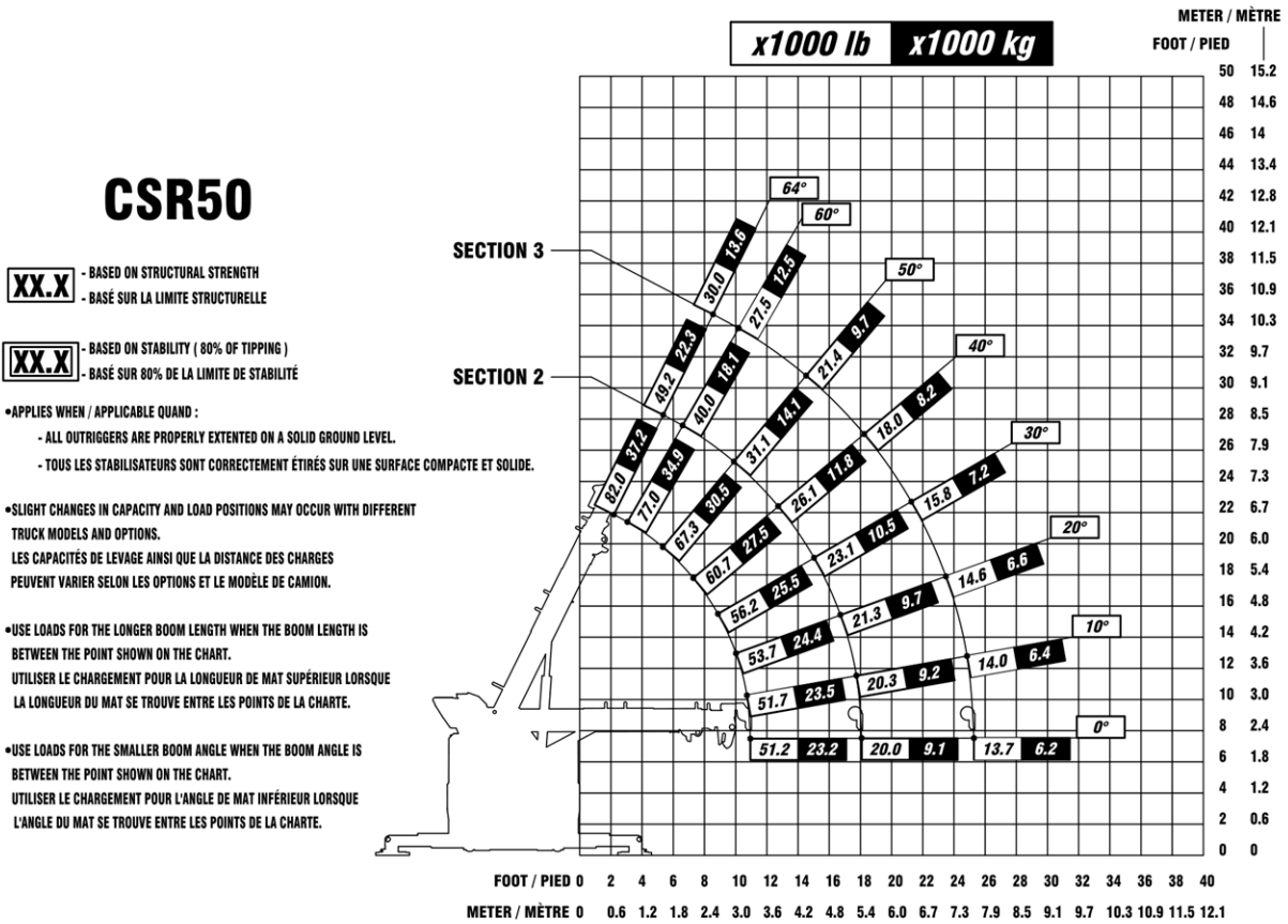
FIGURE 16 – CAPACITÉ DE LEVAGE DU MODÈLE CSR50 À PARTIR DU CÔTÉ
