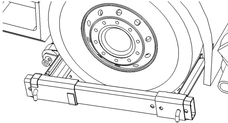
FIGURE 71 – INSTALLER LES COURROIES
