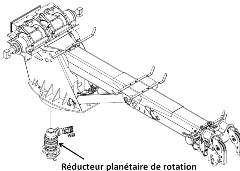
FIGURE 41 – EMPLACEMENT DU RÉDUCTEUR PLANÉTAIRE DE ROTATION
