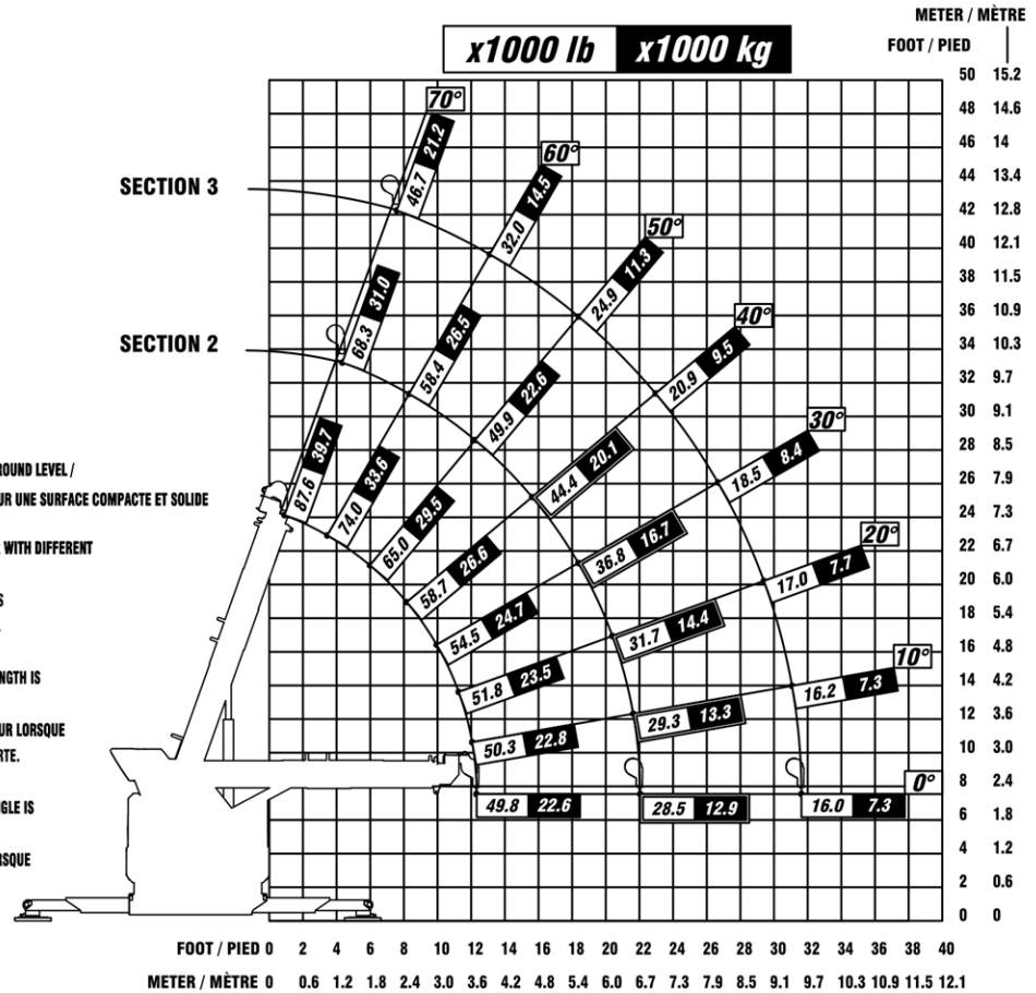
FIGURE 18 – CAPACITÉ DE LEVAGE DU MODÈLE CSR65 À PARTIR DU CÔTÉ
