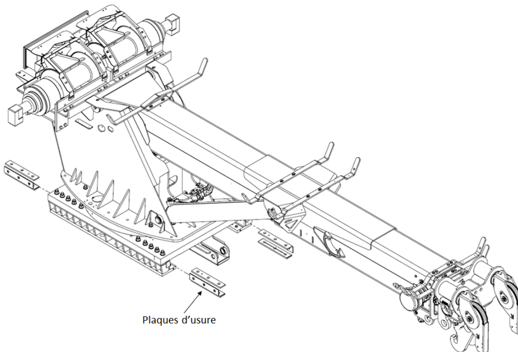
FIGURE 39 – PLAQUES D'USURE – SYSTÈME COULISSANT
