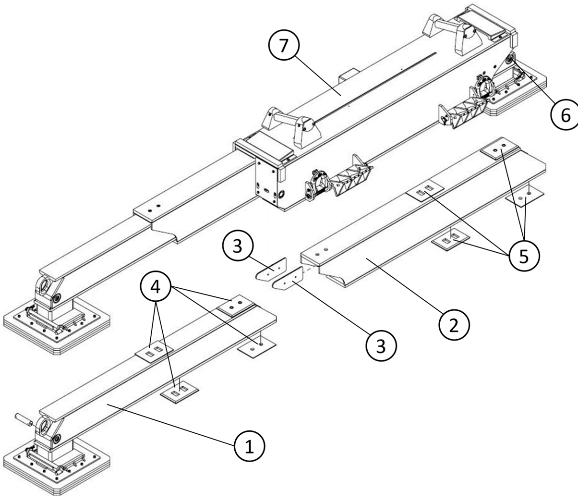
FIGURE 61 – DÉMONTER LE STABILISATEUR (CSR85)
