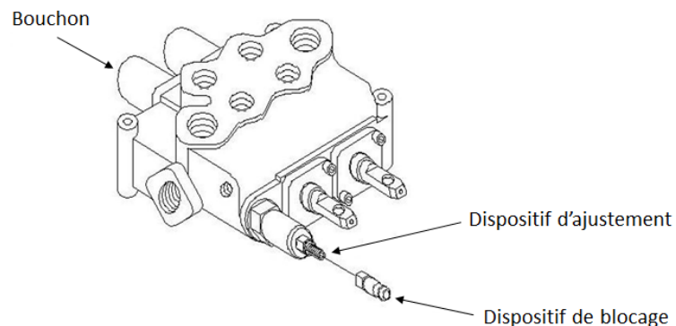
FIGURE 53 – AJUSTER LA PRESSION HYDRAULIQUE SUR LE MODÈLE CSR85 (SOUPAPE DE SURPRESSION PRINCIPALE)
