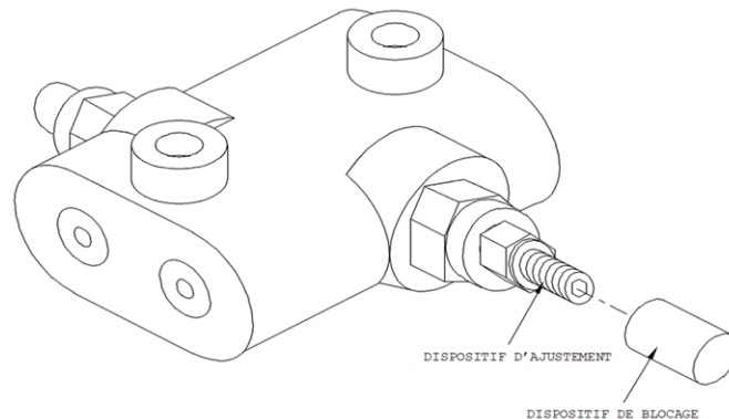
FIGURE 59 – AJUSTEMENT DE LA SOUPAPE D'AMORTISSEMENT
