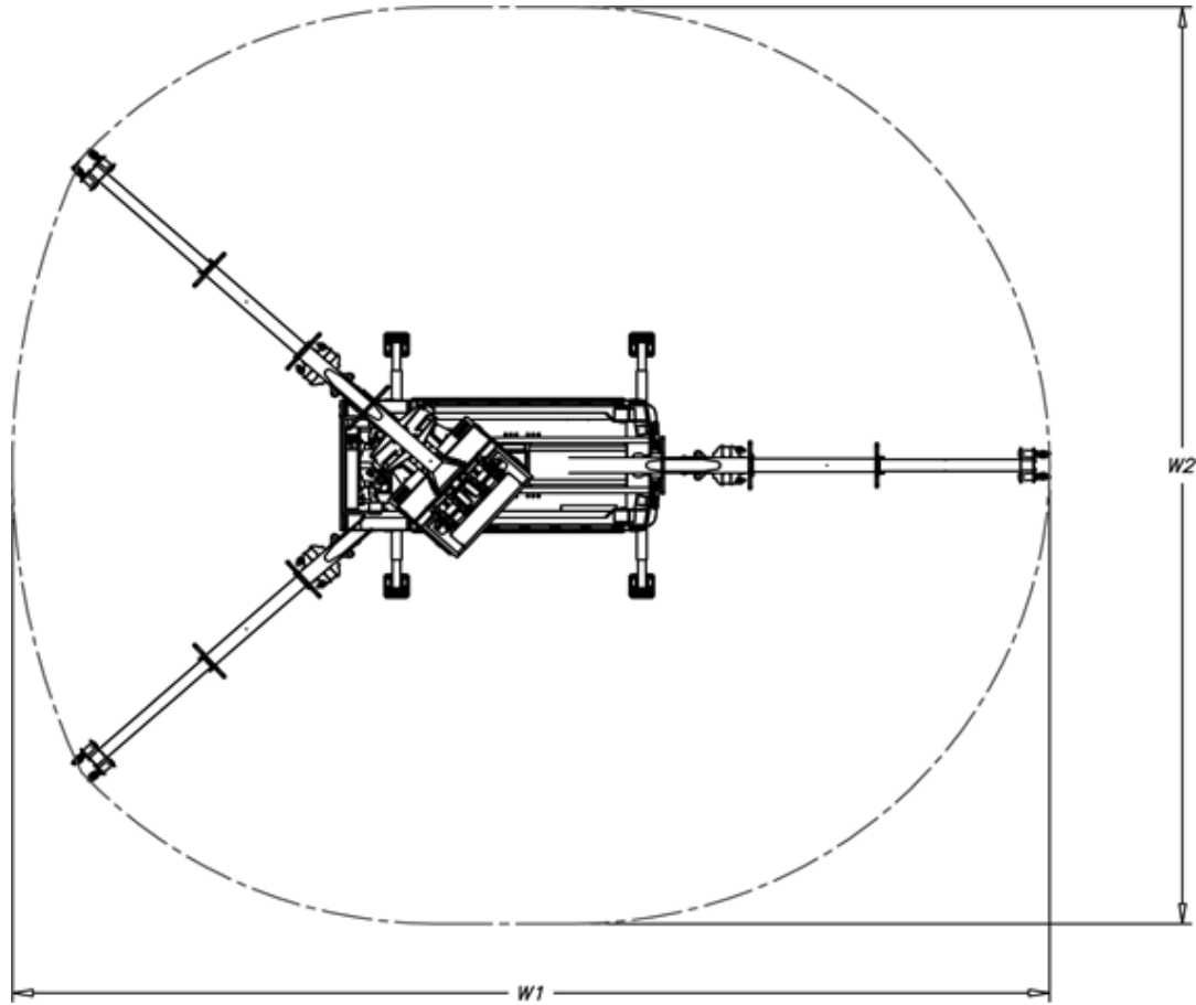
FIGURE 13 – DIMENSIONS DE LA ZONE DE TRAVAIL - VUE DE DESSUS (EXEMPLE)
