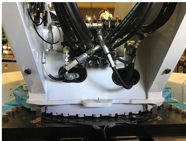
FIGURE 51 – EMBLACEMENT DU DISTRIBUTEUR DANS LA BASE DE LA FLÈCHE (CSR85)
