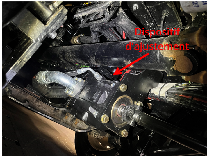
FIGURE 50 – EMBLACEMENT DE LA VIS POUR L'AJUSTEMENT DE LA PRESSION DE LA POMPE HYDRAULIQUE (CSR85)
