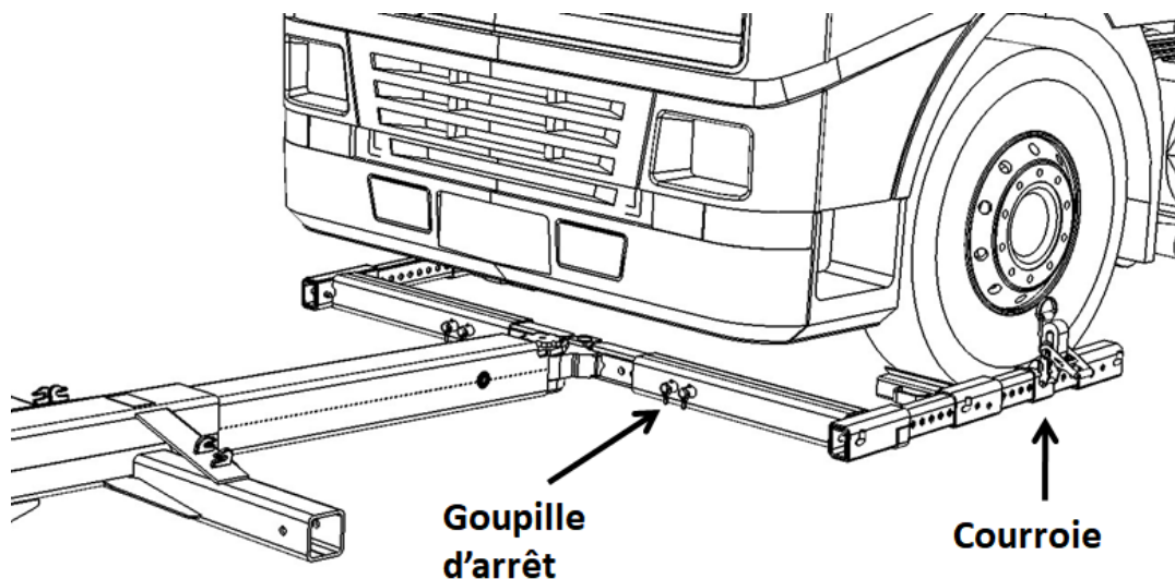
FIGURE 73 – INSTALLER LES LÈVE-PNEUS POUR VÉHICULES DE POIDS MOYEN
