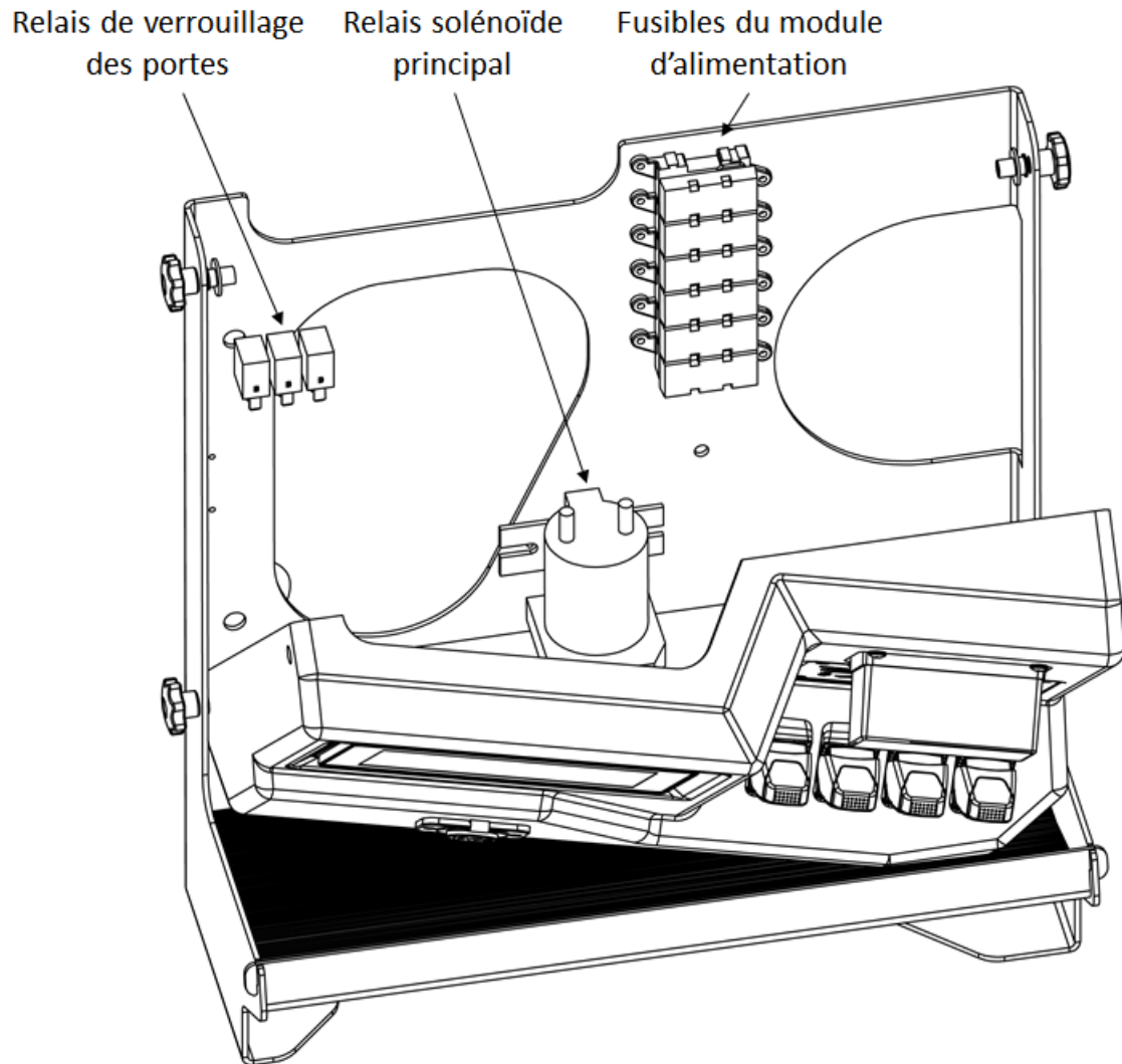
FIGURE 7 – PANNEAU DES ÉCRANS, OUVERT (CÔTÉ GAUCHE) (EXEMPLE)
