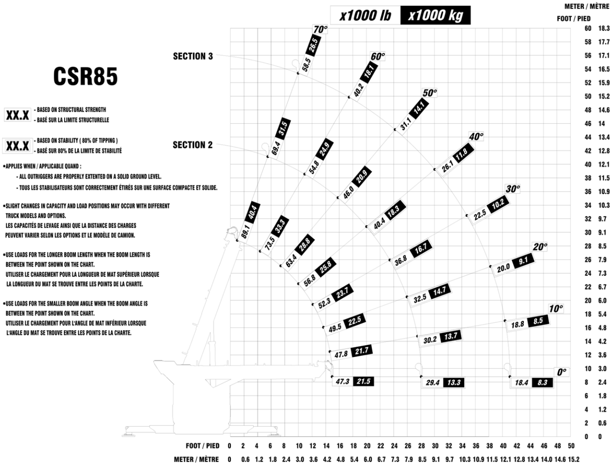
FIGURE 20 – CAPACITÉ DE LEVAGE DU MODÈLE CSR85 À PARTIR DU CÔTÉ
