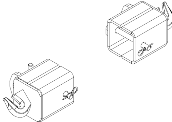
FIGURE 67 – EXEMPLE DE SUPPORTS DE TRAVERSES DE REMORQUAGE
