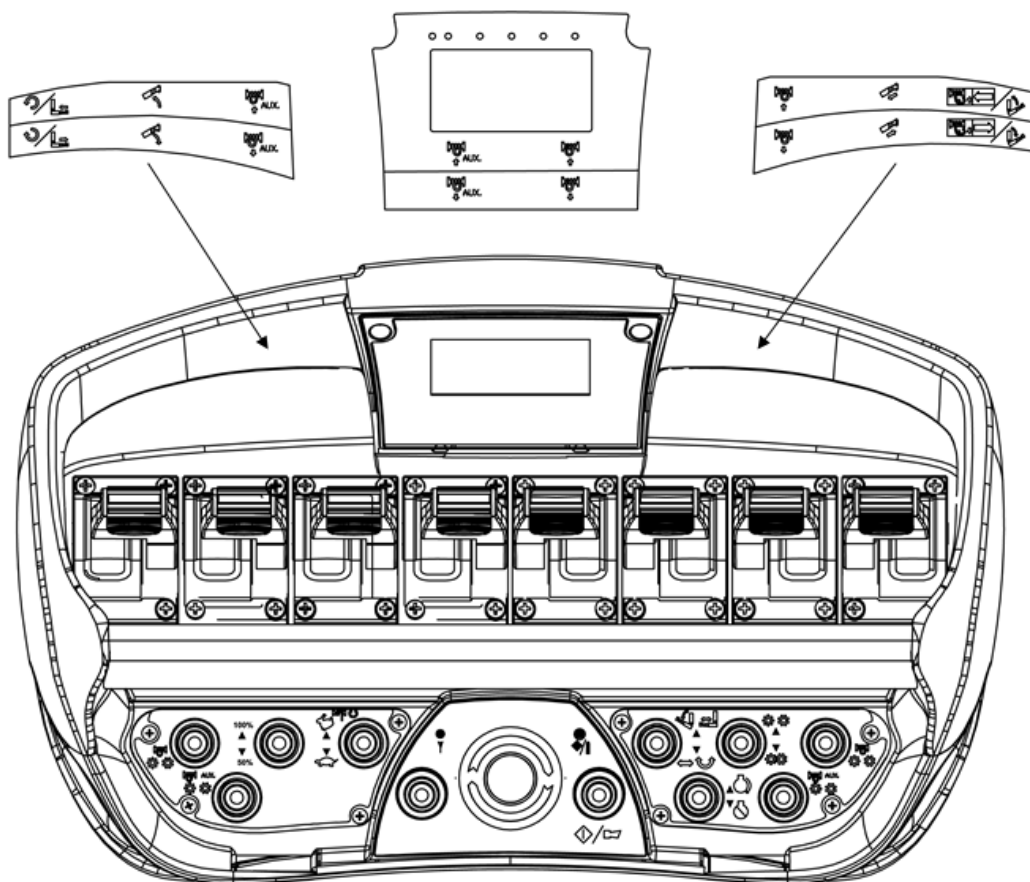
FIGURE 8 – TÉLÉCOMMANDE (EXEMPLE)
