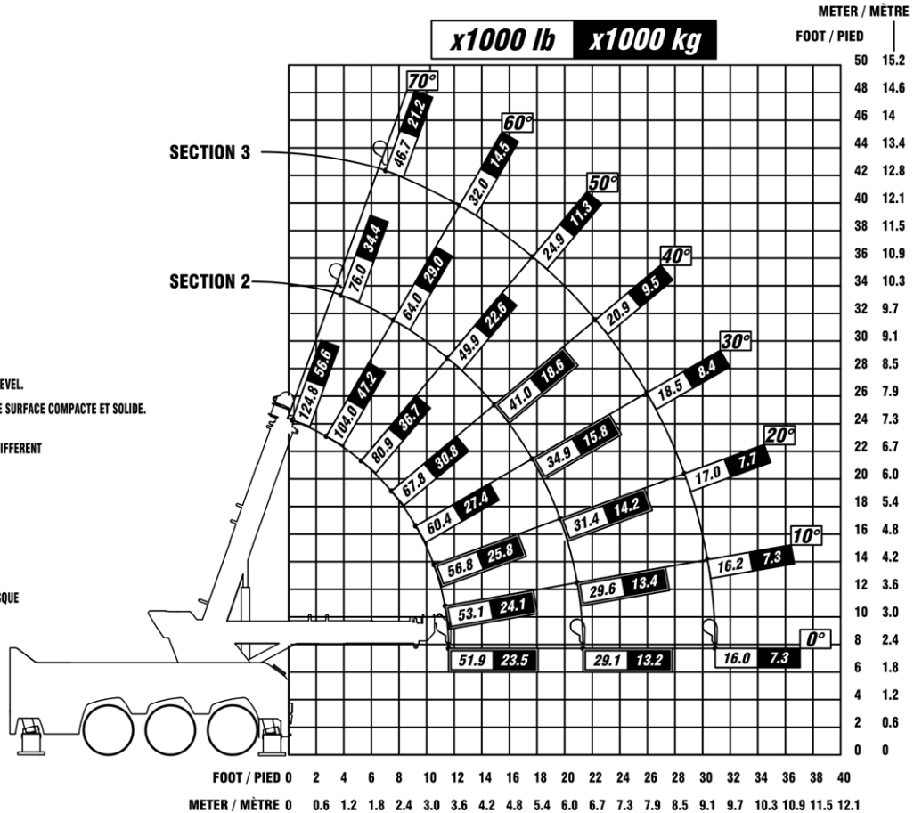
FIGURE 17 – CAPACITÉ DE LEVAGE DU MODÈLE CSR65 À PARTIR DE L'ARRIÈRE
