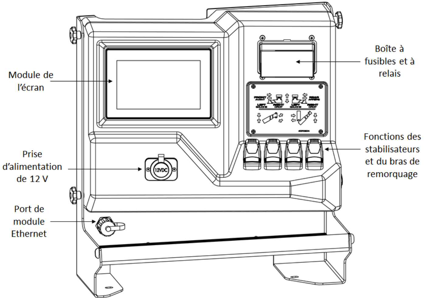
FIGURE 6 – PANNEAU DES ÉCRANS, FERMÉ (CÔTÉ GAUCHE) (EXEMPLE)
