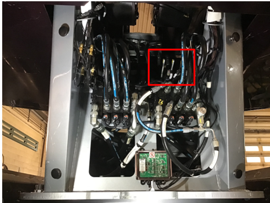
FIGURE 24 – DÉRIVATION HYDRAULIQUE D'URGENCE DANS LA BASE DU SYSTÈME COULISSANT ROTATIF
