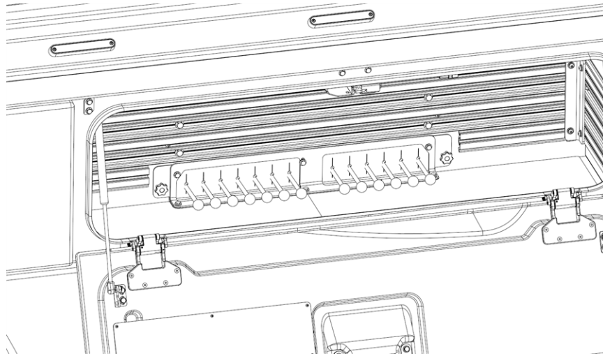
FIGURE 23 – PANNEAU DE COMMANDE DE LA DÉRIVATION HYDRAULIQUE D'URGENCE
