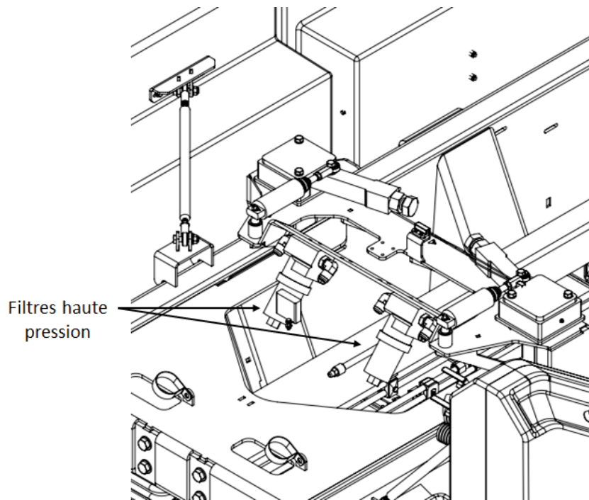
FIGURE 42 – FILTRES À HAUTE PRESSION – CSR50
