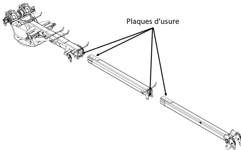
FIGURE 37 – PLAQUES D'USURE – FLÈCHE
