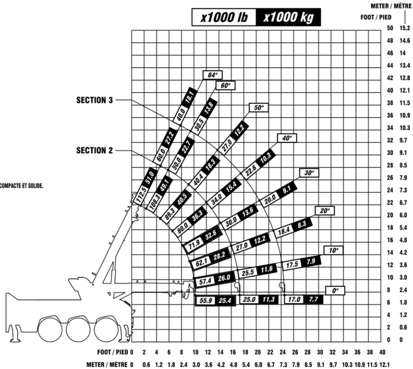
FIGURE 15 – CAPACITÉ DE LEVAGE DU MODÈLE CSR50 À PARTIR DE L'ARRIÈRE
