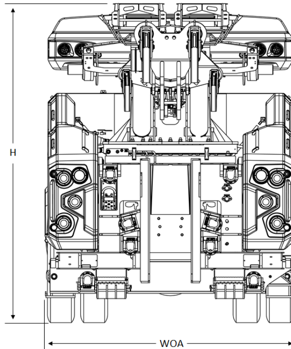
FIGURE 10 – DIMENSIONS DU CHÂSSIS - VUE DE DESSUS (EXEMPLE)
