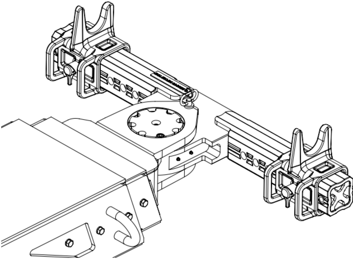
FIGURE 66 – EXEMPLE DE SUPPORTS À FOURCHES INTÉGRÉES
