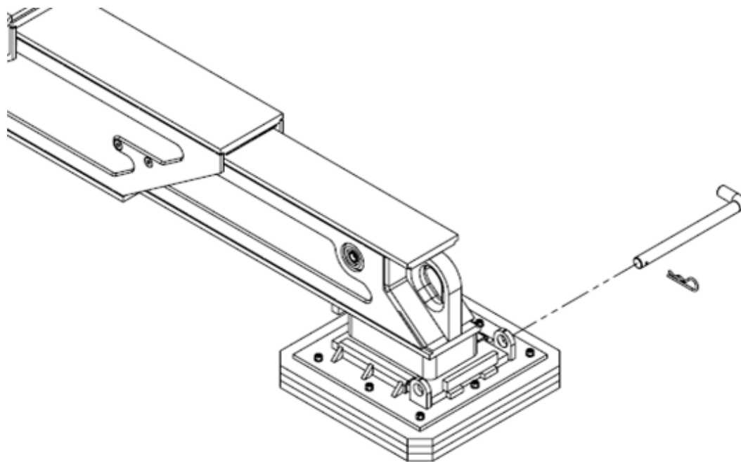
FIGURE 79 – INSTALLER LES PLAQUES DE BOIS
