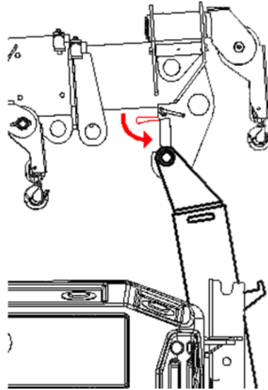
FIGURE 27 – DÉVERROUILLER L'ATTACHE DE SÉCURITÉ (EXEMPLE)
