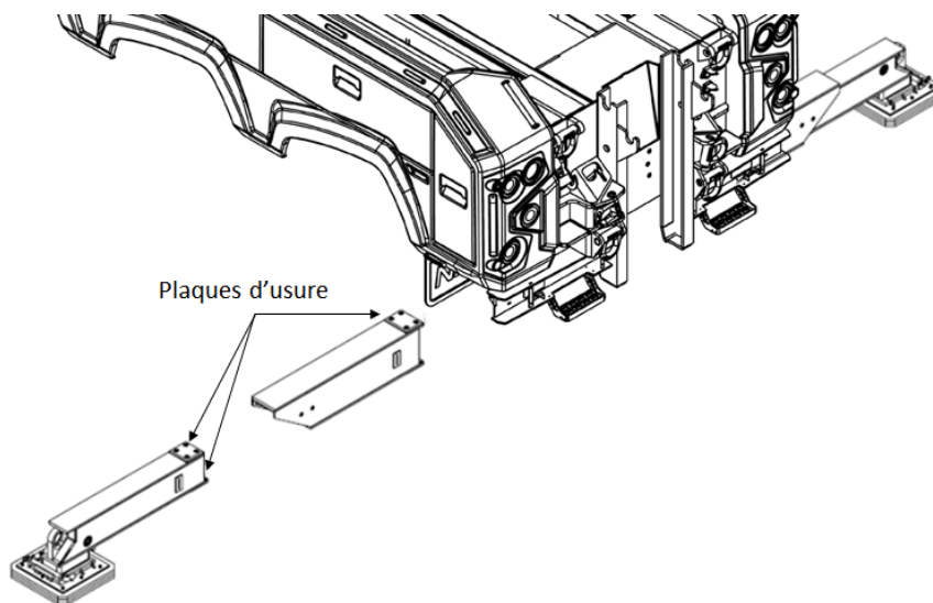
FIGURE 38 – PLAQUES D'USURE – STABILISATEURS
