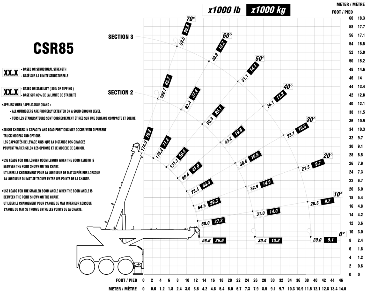
FIGURE 19 – CAPACITÉ DE LEVAGE DU MODÈLE CSR85 À PARTIR DE L'ARRIÈRE
