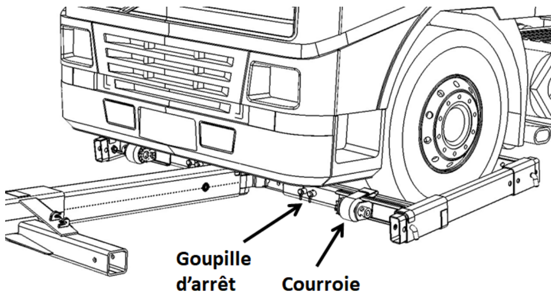
FIGURE 70 – INSTALLER LES LÈVE-PNEUS POUR VÉHICULES LOURDS SUR LA TÊTE DE LA TRAVERSE DE REMORQUAGE
