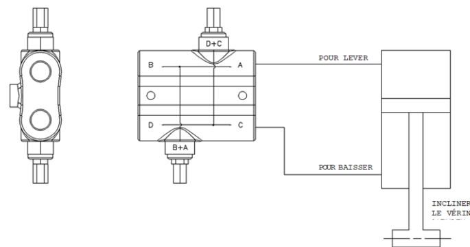
FIGURE 58 – AJUSTEMENT DE LA SOUPAPE D'AMORTISSEMENT DU BRAS DE REMORQUAGE
