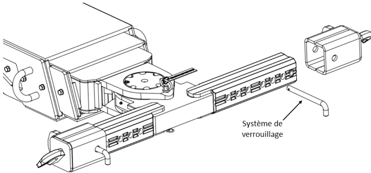
FIGURE 68 – INSTALLER LES SUPPORTS DE TRAVERSES DE REMORQUAGE
