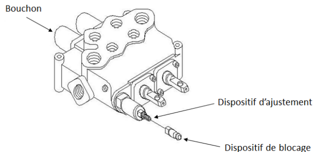
FIGURE 49 – AJUSTER LA PRESSION HYDRAULIQUE SUR LES MODÈLES CSR50 ET CSR65 (SOUPAPE DE SURPRESSION PRINCIPALE)
