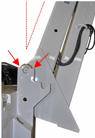
FIGURE 31 – PLACER LE BRAS DE REMORQUAGE DANS LES RAILS (EXEMPLE)
