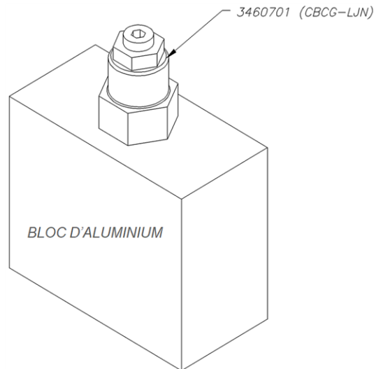
FIGURE 54 – AJUSTER UNE SOUPE D'ÉQUILIBRAGE (CBCG-LJN)
